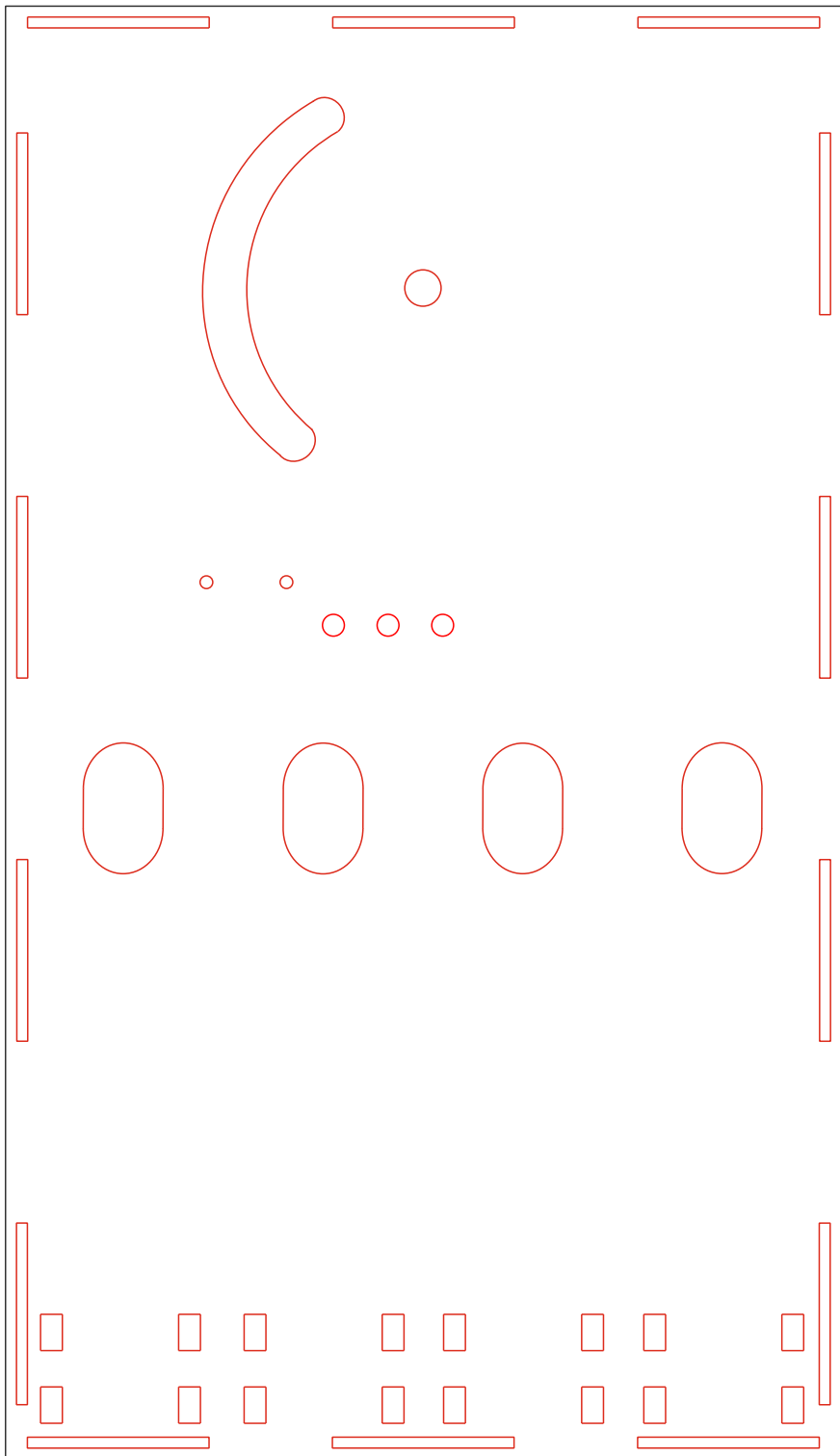
Donja ploča postolja
