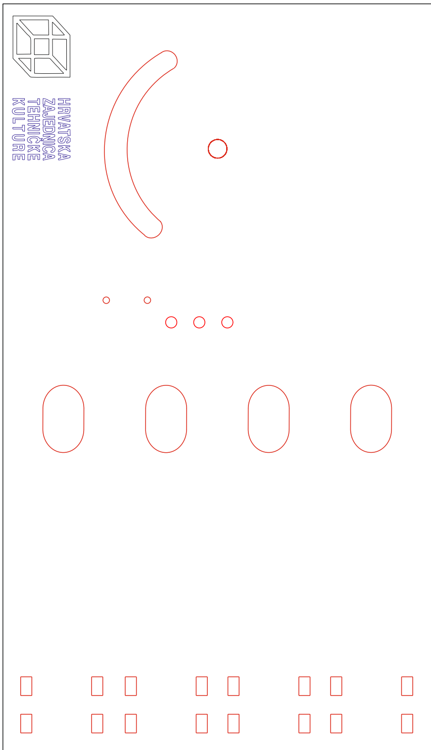
Gornja ploča postolja
