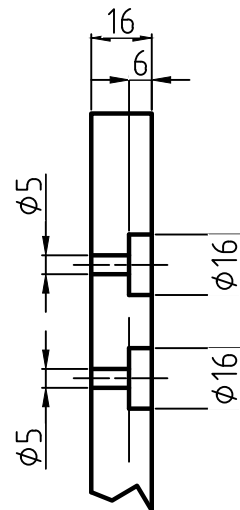
PRESJEK A-A
